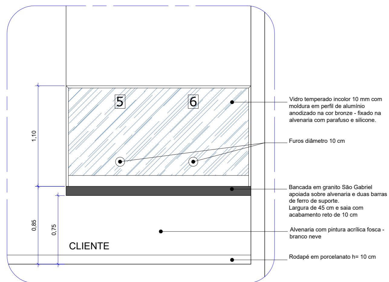
04 SITUAÇÃO FUTURA - VISTA Esc.: 1/25
