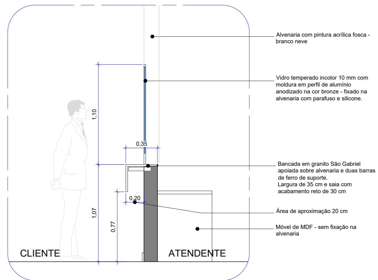
02 SITUAÇÃO ATUAL - CORTE Esc.: 1/25
