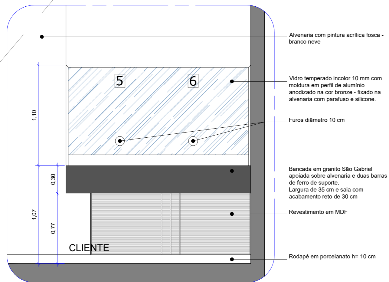
01 SITUAÇÃO ATUAL - VISTA Esc.: 1/25
