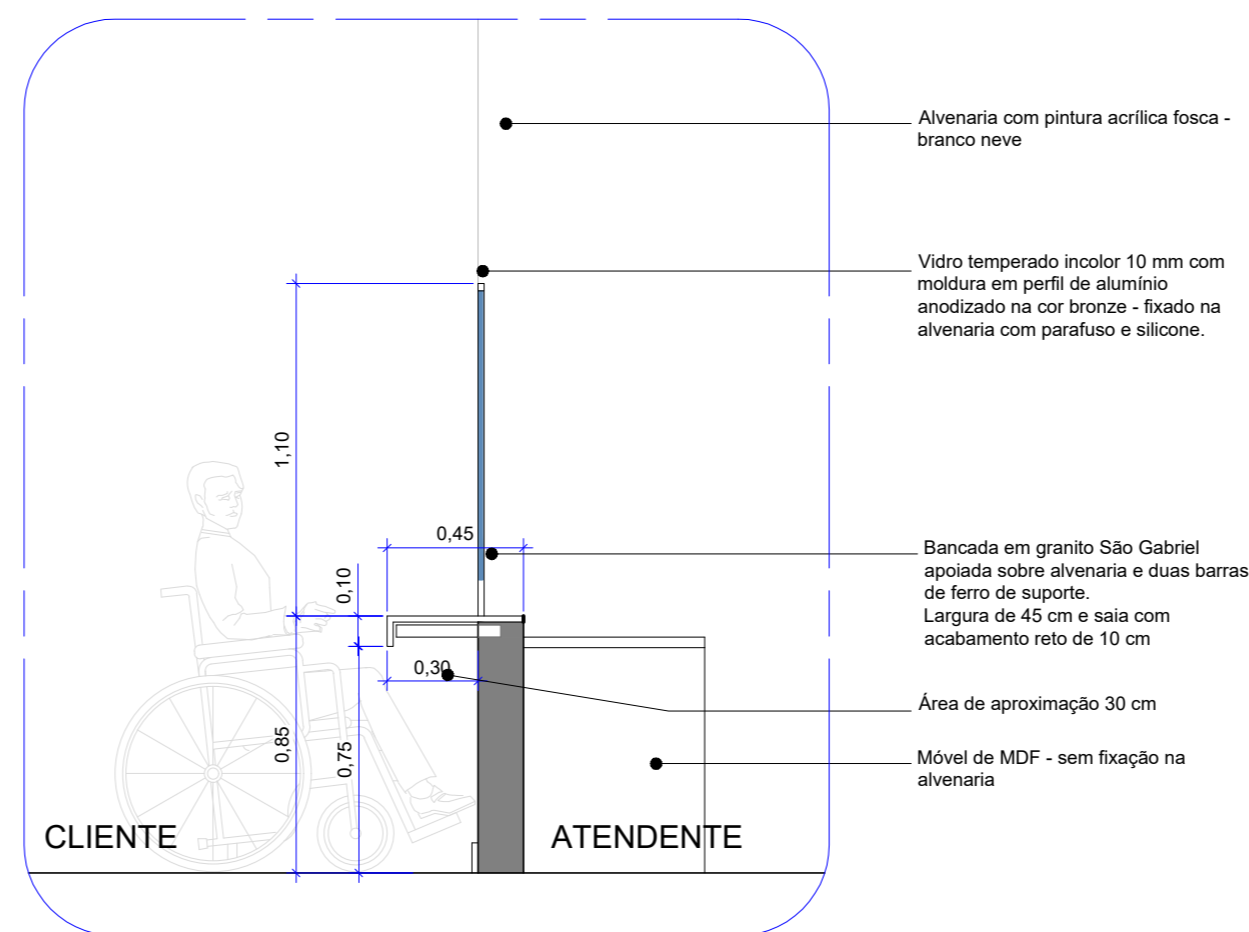
05 SITUAÇÃO FUTURA - CORTE Esc.: 1/25
