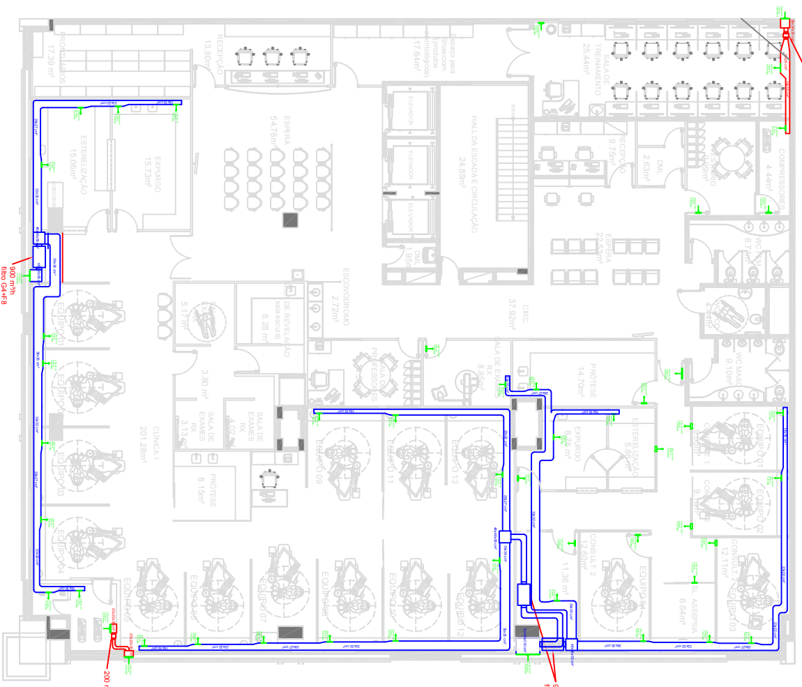
01 PLANTA DE LOCAÇÃO DOS DUTOS E EQUIPAMENTOS Esc. 1100
